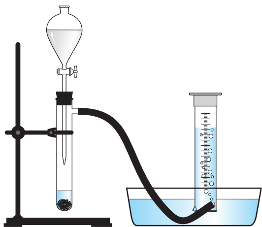
Skābekļa iegūšana, izspiežot ūdeni
