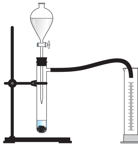
Skābekļa iegūšana, izspiežot gaisu
