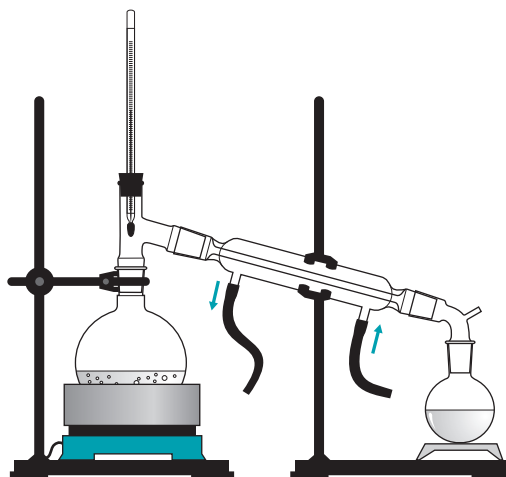
Destilācija
